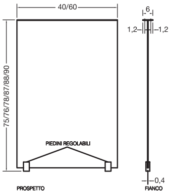
Disegno tecnico acciaio Technical drawer of steel finish
