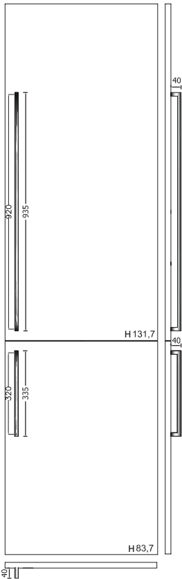
ANTA CESTELLO ESTRAIBILE PULL-OUT BASKET DRAWER DOOR
