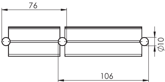
VISTA SUPERIORE TOP VIEW
