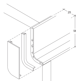
Passante fianco terminale anta base / Single horizontal c-shaped groove placed on end side panel / Горизонтальная одиночная изогнутая Gola на боковине.
