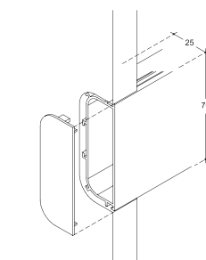
Passante fianco terminale cestoni base / Double horizontal flat groove placed on end side panel / Горизонтальная двойная плоская Gola на боковине.
