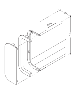
Passante fianco terminale cestoni base / Double horizontal c-shaped groove placed on end side panel / Горизонтальная двойная изогнутая Gola на боковине.
