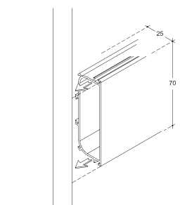
Battuta fianco terminale cestoni base / Double horizontal flat groove leaned against end side panel / Горизонтальная двойная плоская Gola до боковины.
