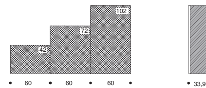
PENSILE - ANTA VETRO SERIGRAFATO / WALL UNIT - SERIGRAPHY GLASS DOOR / НАВЕСНЫЙ ШКАФ - ДВЕРЬ СО СЕРИГРАФИРОВАННЫМ СТЕКЛОМ
