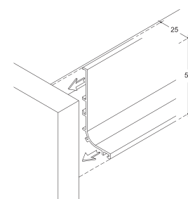
Battuta fianco terminale anta base / Single horizontal c-shaped groove leaned against end side panel / Горизонтальная одиночная изогнутая Gola до боковины.
