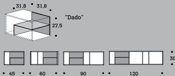
PENSILE A GIORNO "JUMPY" + "DADO" "JUMPY" + "DADO" OPEN WALL UNITS ÉLÉMENTS HAUTS SOSPENSUS OUVERTS "JUMPY" + "DADO" Orizzontale
